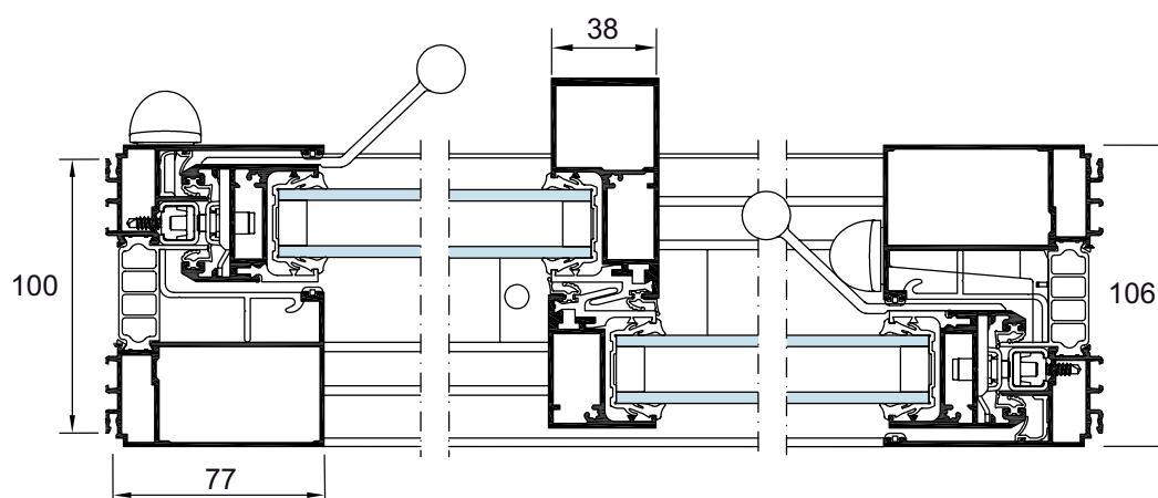
Sección horizontal
