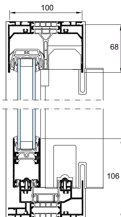
Sección vertical
