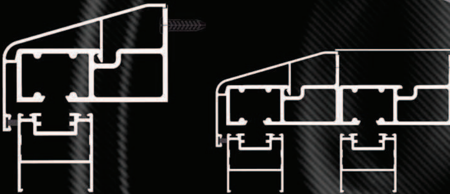
Opciones guía inferior (también sin guía inferior con ángulo de acero + guiador)
