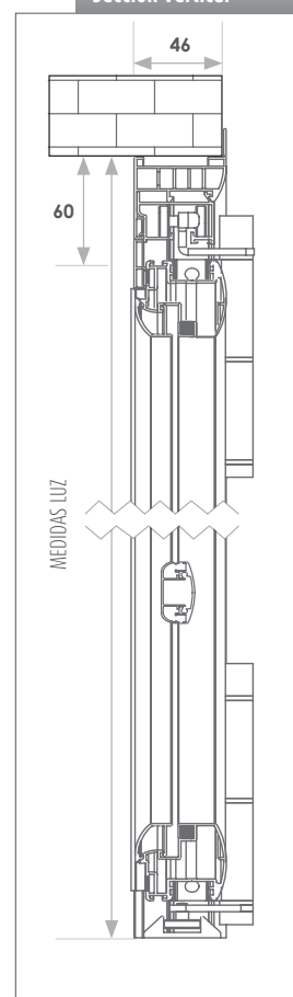
Sección vertical
