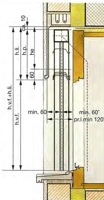
Sección vertical. Montaje detrás del dintel. Pueden estudiarse otros modelos de montaje.
